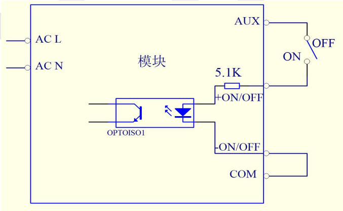
图 4 遥控接线图
