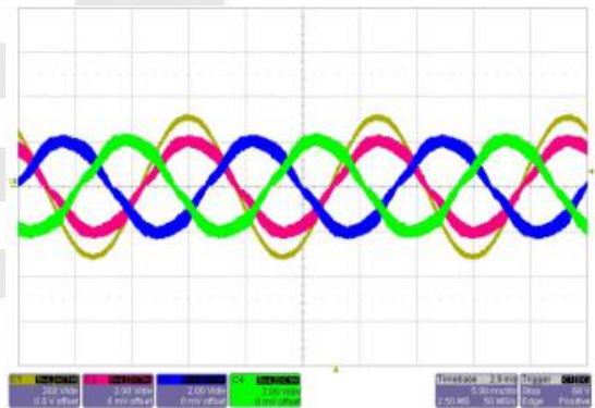
图 6: 半载情况下典型输入电流波形(1000W)
