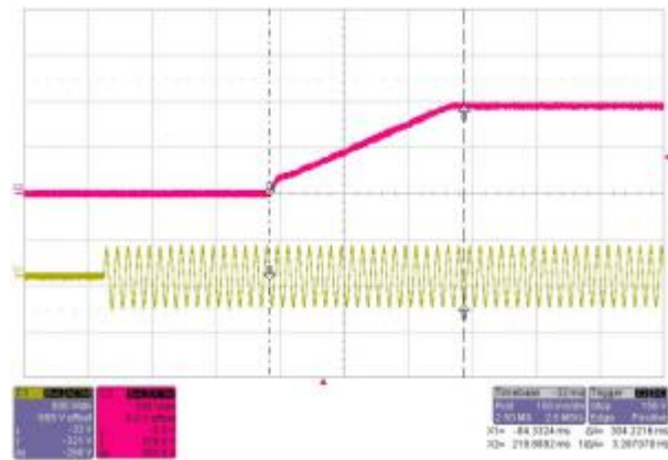
图 8: 半载情况下启机波形 (1000W)
