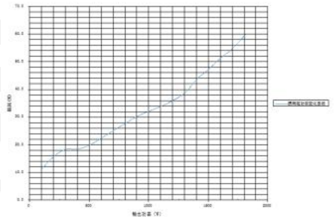
图 2: 功率损耗 vs. 输出功率曲线 (30°C 基板温度)
