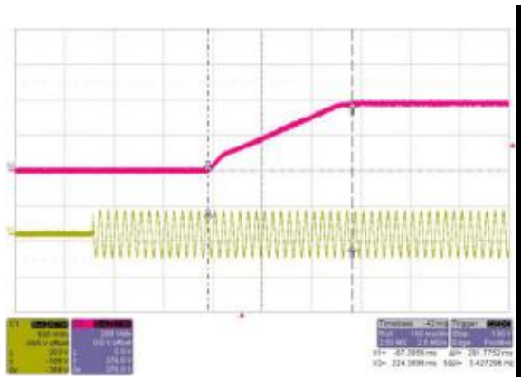
图 7: 满载条件下启机波形(2000W)
