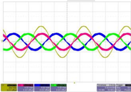
图 5: 满载条件下典型输入电流波形(2000W)
