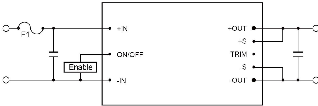
模块运行示意图
